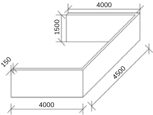
Figur 1 Figur 1 er 3D-tegningen til de vægge/sider, der skal støbes.
